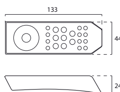
Remote (S3.10.0424)
