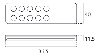
Remote (S3.10.0474)
