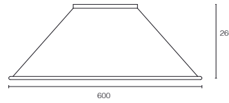
Reflector Alu. 100°
