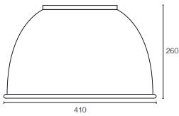
Reflector PC 80°
